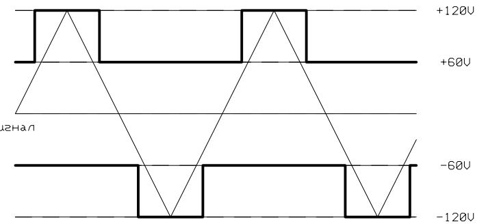
Зависимость отрицательного напряжения питания от выходного сигнала
