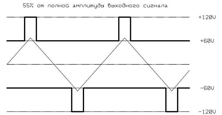
Зависимость отрицательного напряжения питания от выходного сигнала
