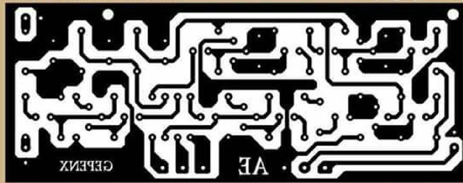
PCB 11,5 x 4,5 cm
